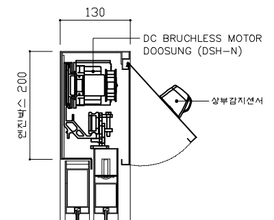
ENGINE BOX 상세도
