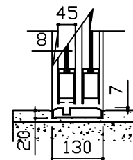
BOTTOM RAIL 문힘 상세도
